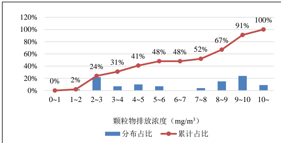
图 5-2 颗粒物排放数据累计分布情况
