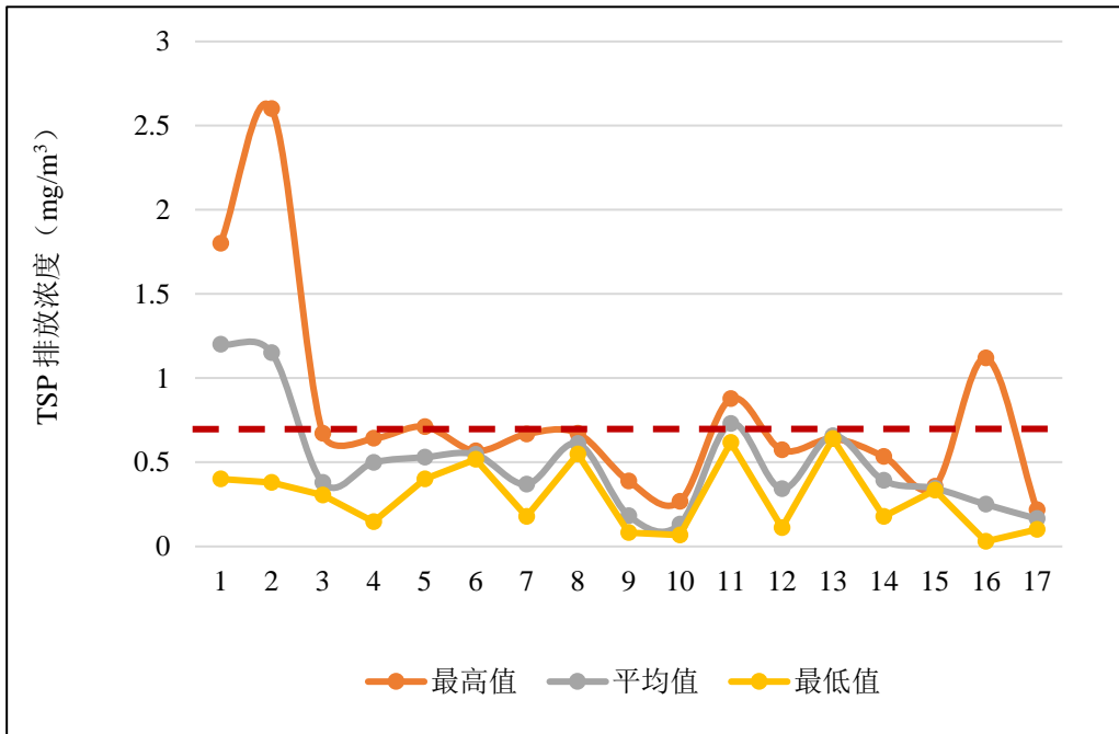
图 5-13 总悬浮颗粒物排放情况
