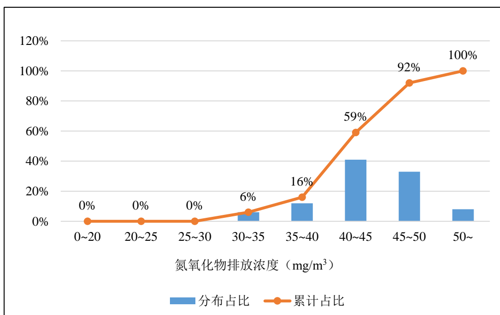
图 5-8 氮氧化物排放数据累计分布情况
