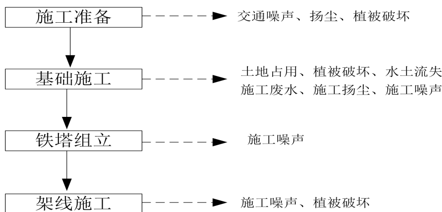
图 19 输电线路建设流程及产污环节示意图
