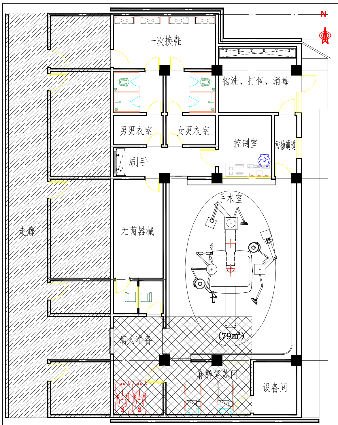
图 1-4 拟建数字减影血管造影室所在楼一层平面设计图
