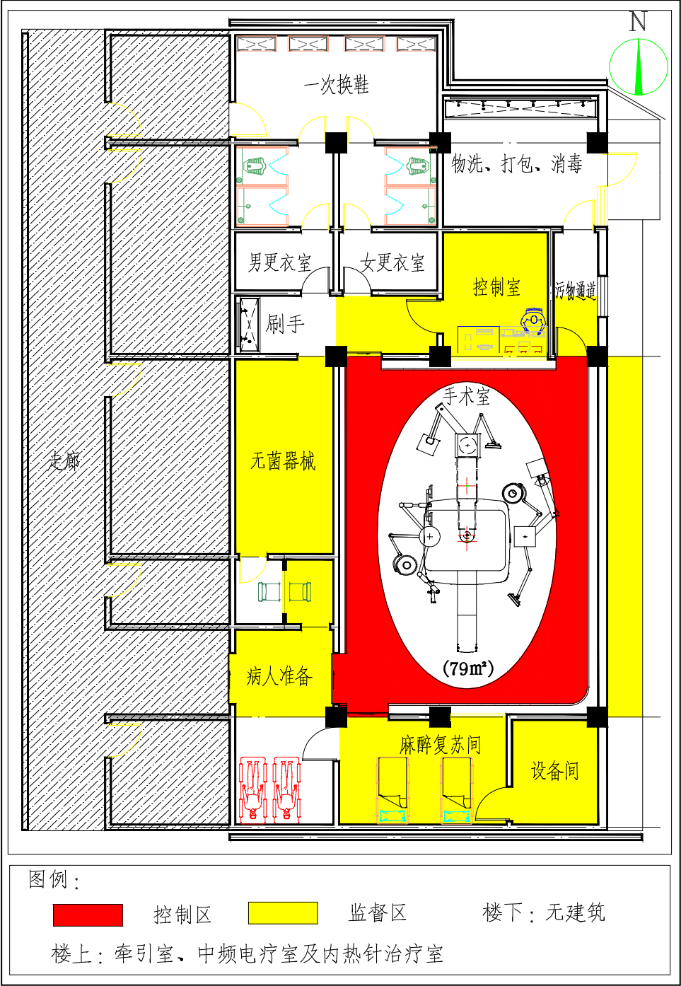
图 10-1 拟建 DSA 机房分区设计图
