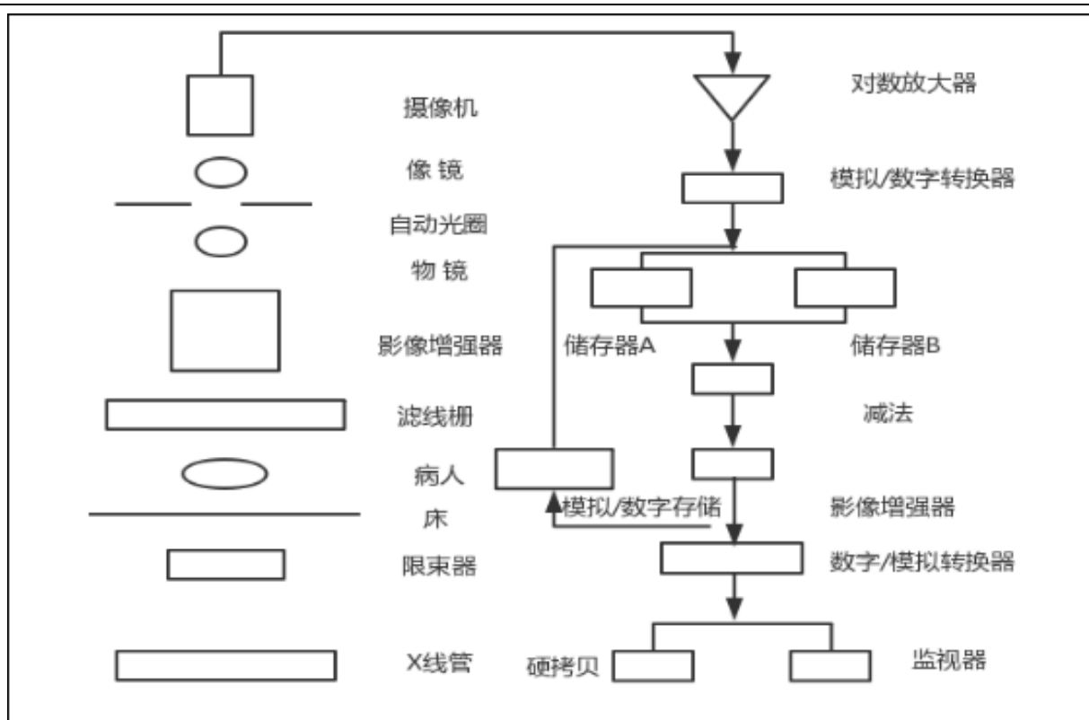
图 9-2 DSA 的设备结构图
