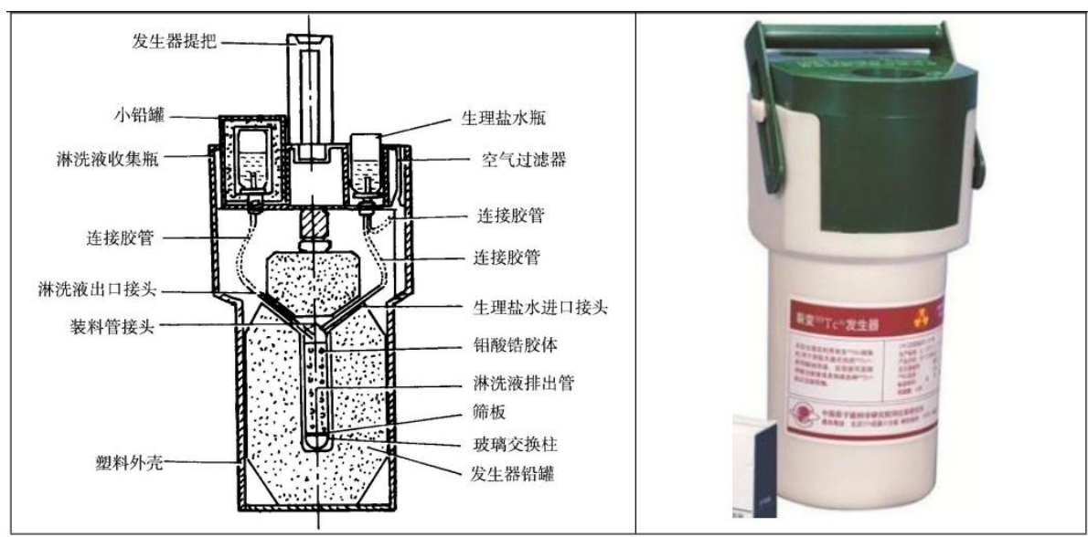
图9-1 99 Mo- 99m Tc发生器的结构示意图
