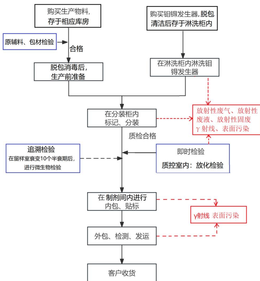
图9-2 ^{99m}\text{Tc} 放射性药物生产工艺流程及产污环节
