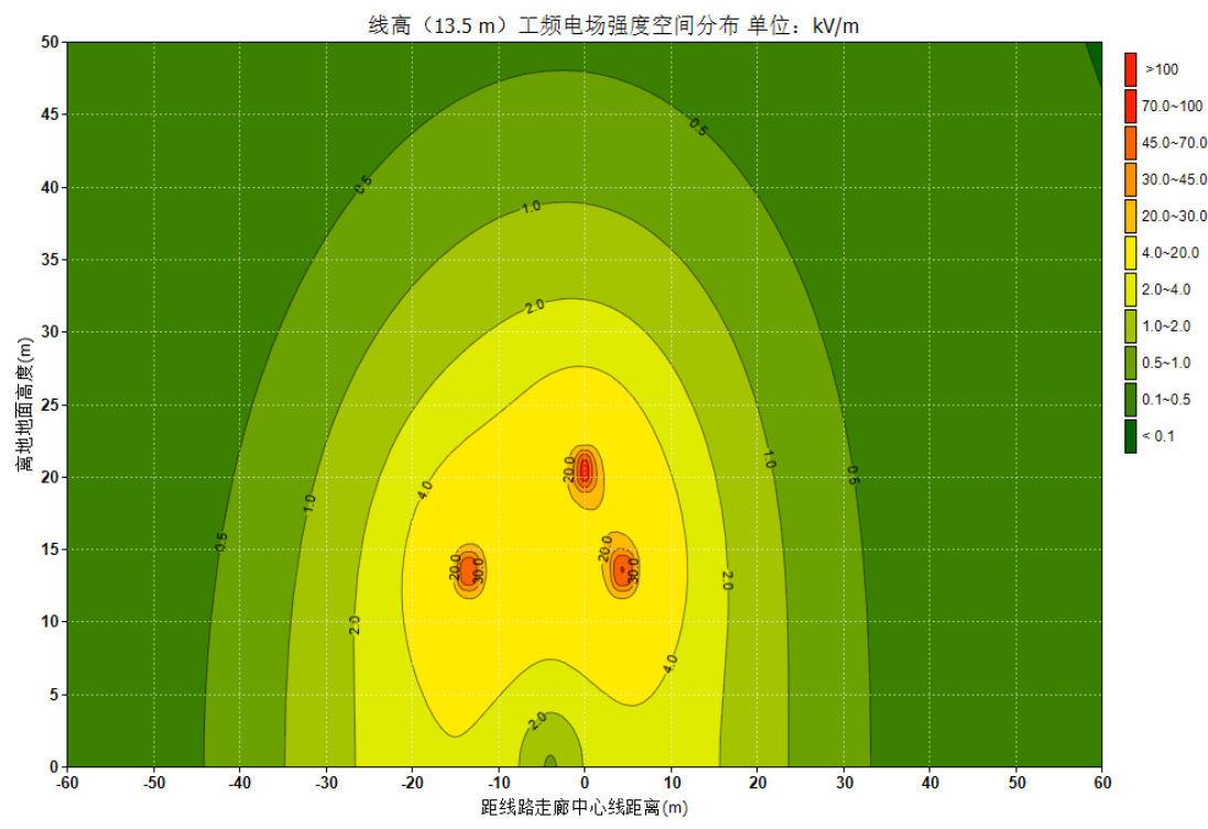
图 6.1-8 新建 330kV 单回线路（三角排列）4kV/m 等值线图
