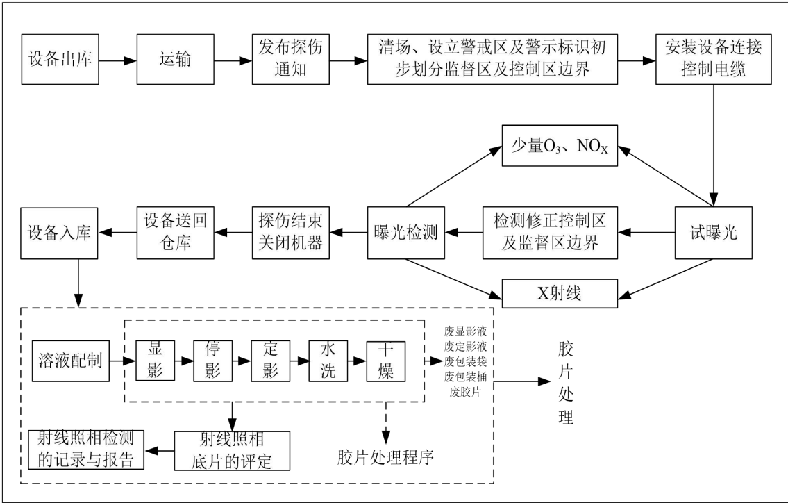
图 9-4 X 射线探伤机移动探伤工艺流程及产污环节示意图
