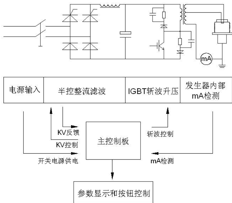
图 9-1 整机电器原理框图
