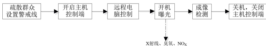
图 9-5 本项目 X 射线探伤装置工作流程及产污环节示意图
