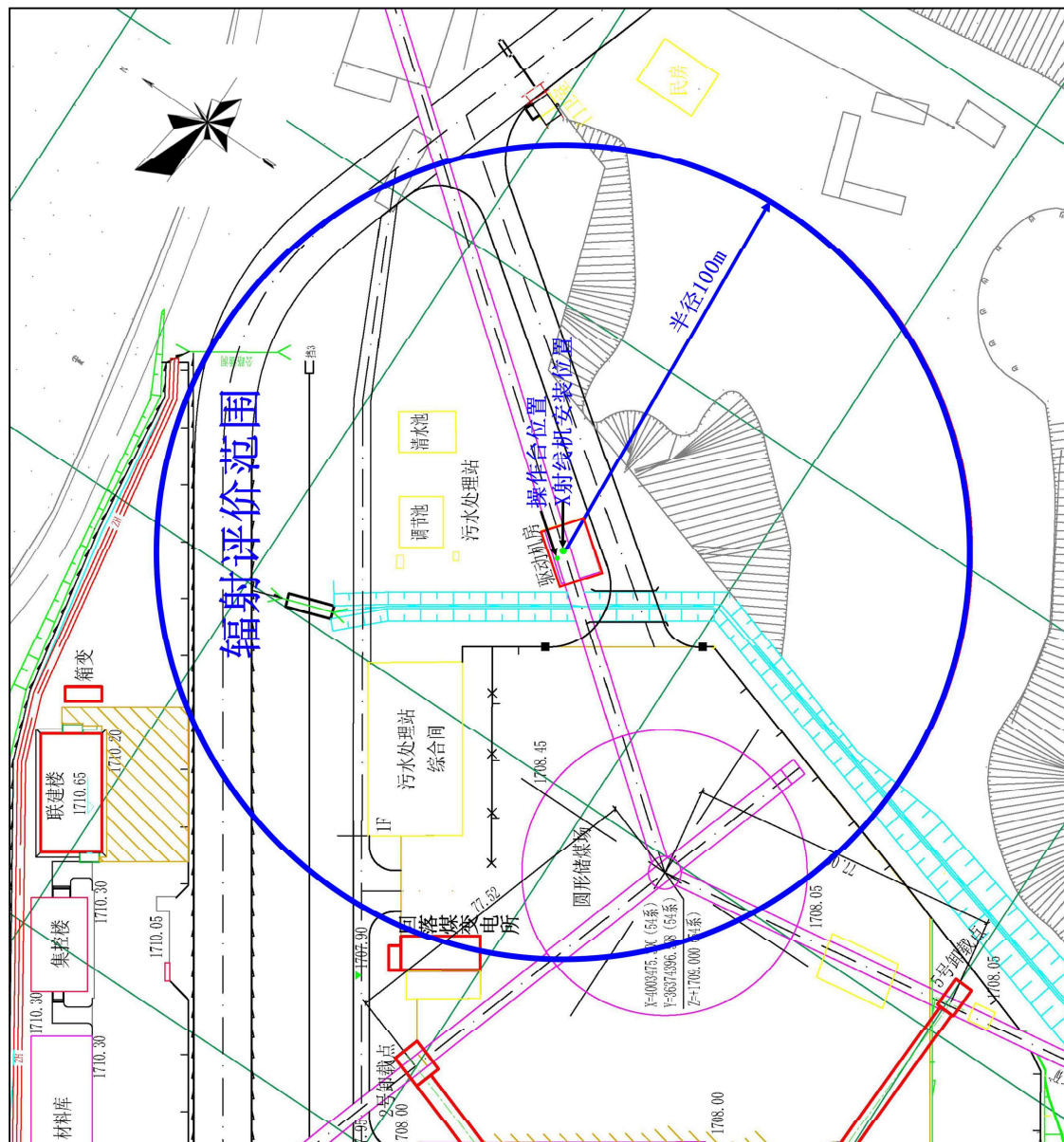
图 1-3 运煤隧道 X 射线探伤装置周边环境及评价范围示意图
