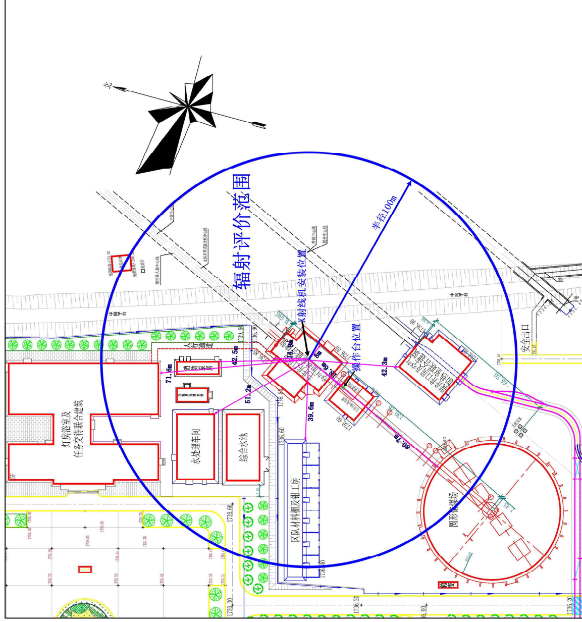
图 11-1 主井井口房及空气加热室联合建筑 X 射线探伤装置周围关注点示意图
