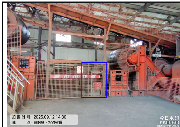
主井井口房及空气加热室联合建筑内 X 射线机安装位置（设置 1.5m 高防护网）
