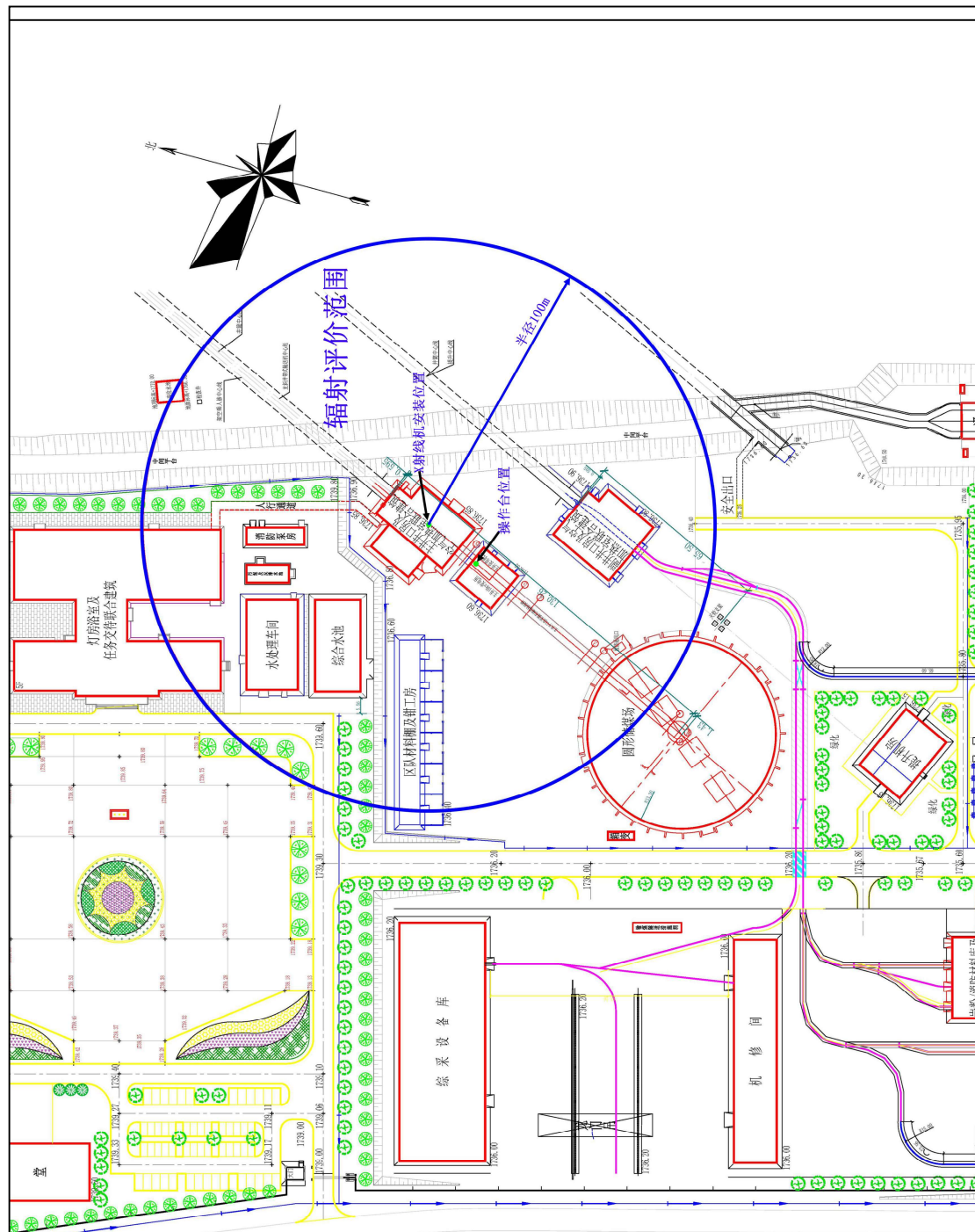
图 1-2 主井井口房及空气加热室联合建筑 X 射线探伤装置周边环境及评价范围示意图
