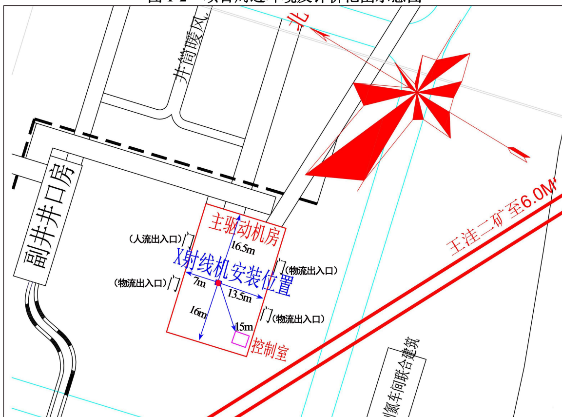
图 1-3 射线装置安装示意图
