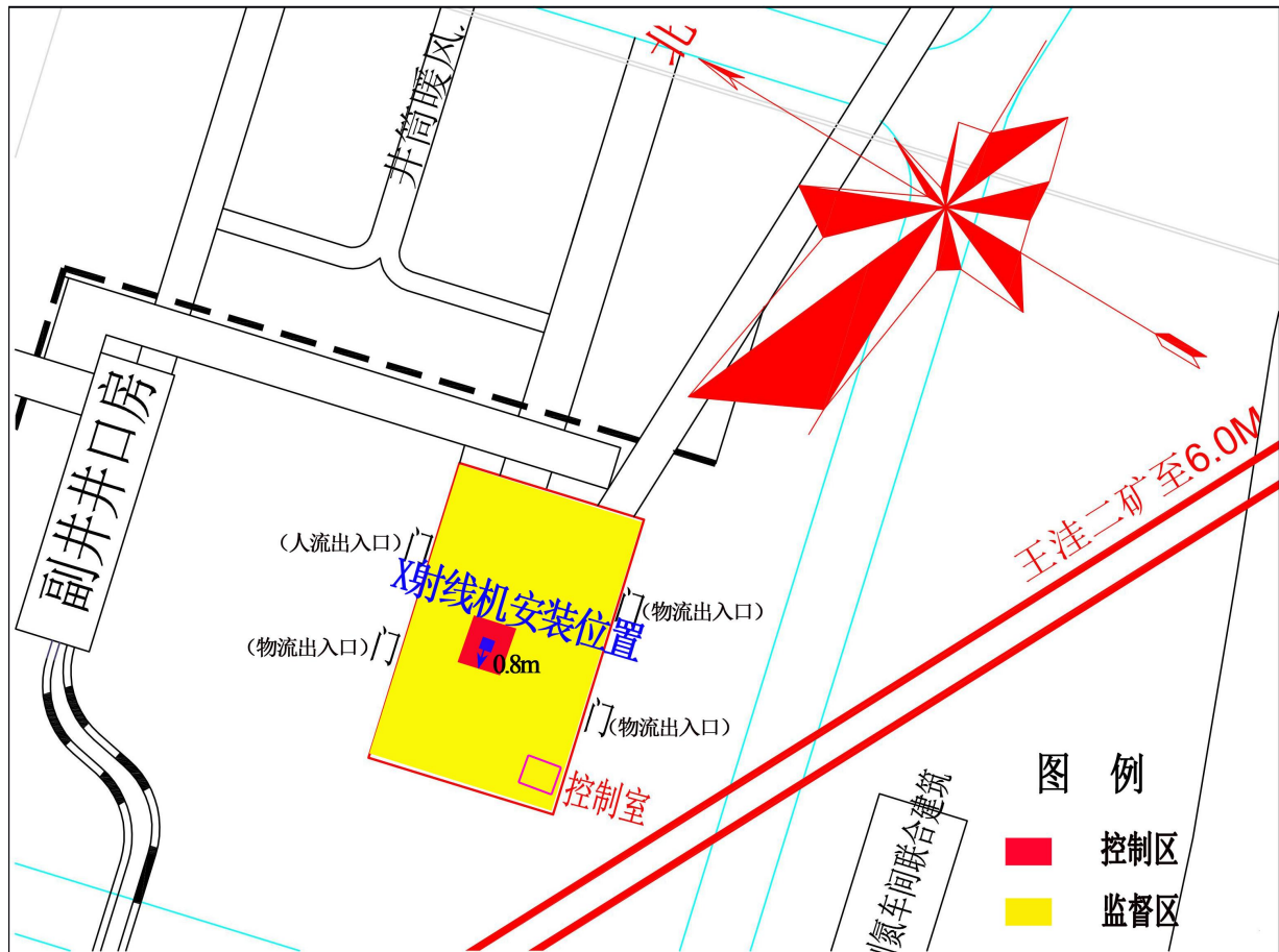
图 10-1 X 射线探伤机控制区和监督区划分示意图
