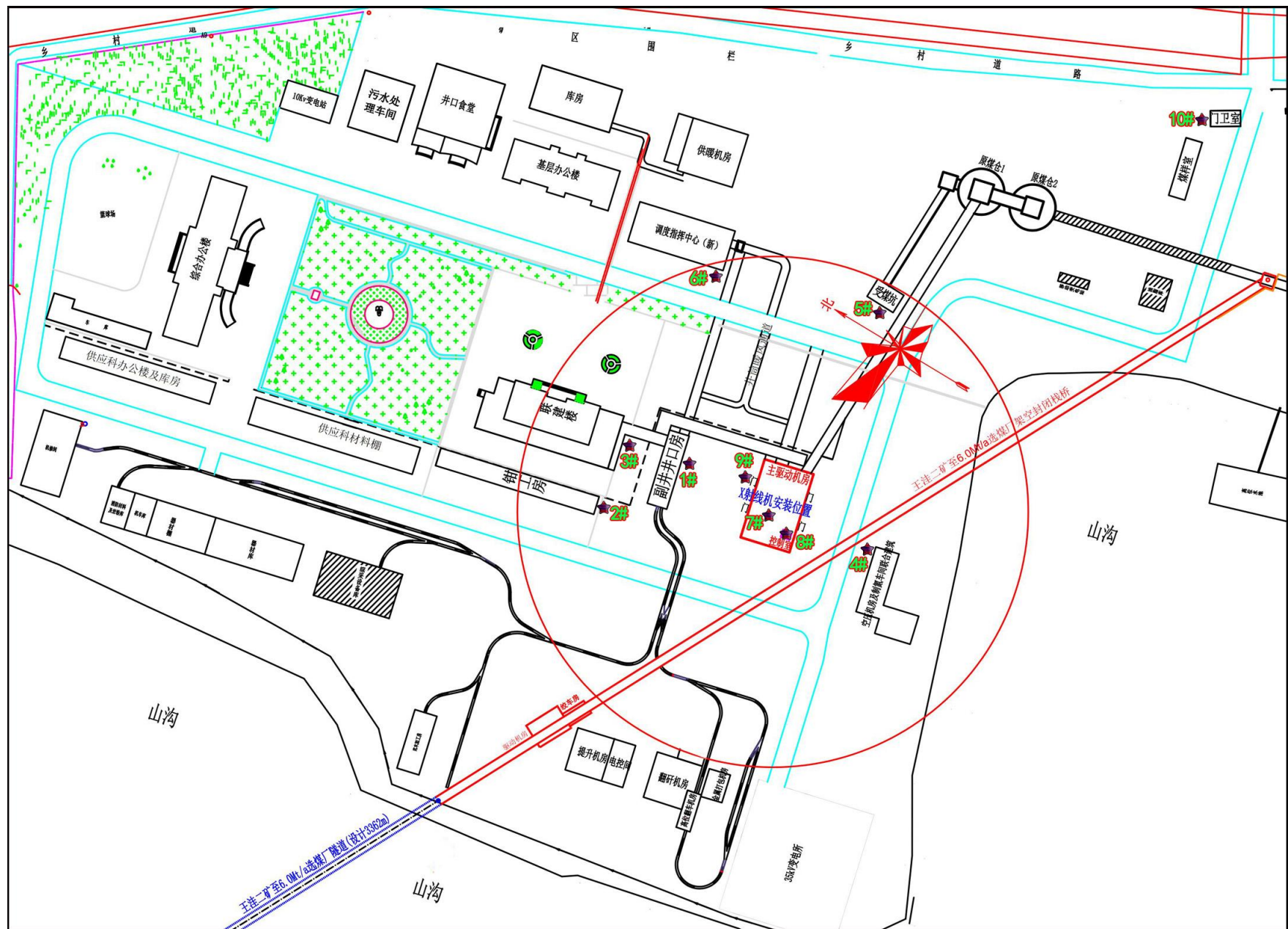
图 8-1 项目 \gamma 辐射瞬时剂量率监测布点图
