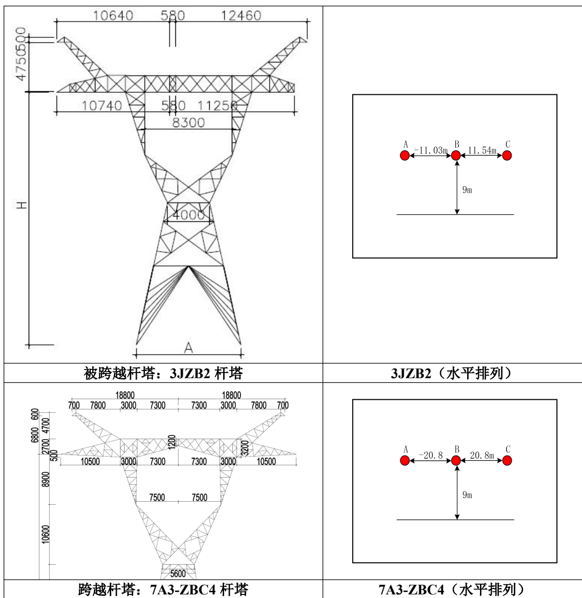
图 6.1-15 本项目交叉跨越预测选取的塔型
