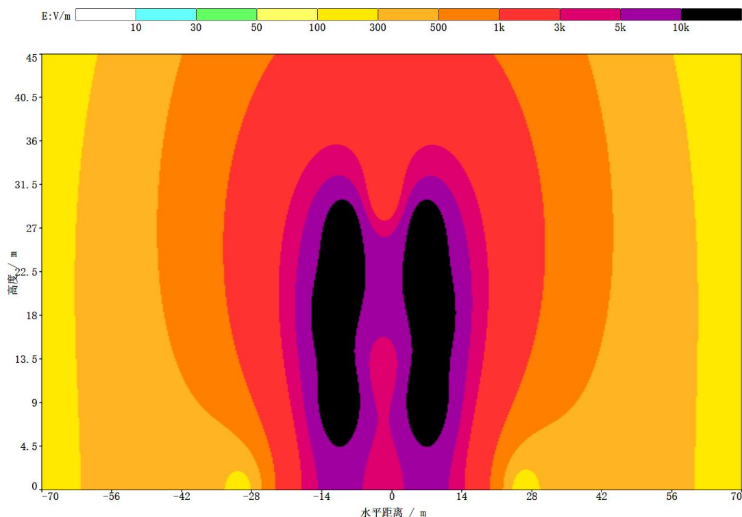
图 6.1-10 新建 330\text{kV} 双回线路（双侧挂线） 4\text{kV/m} 等值线图
