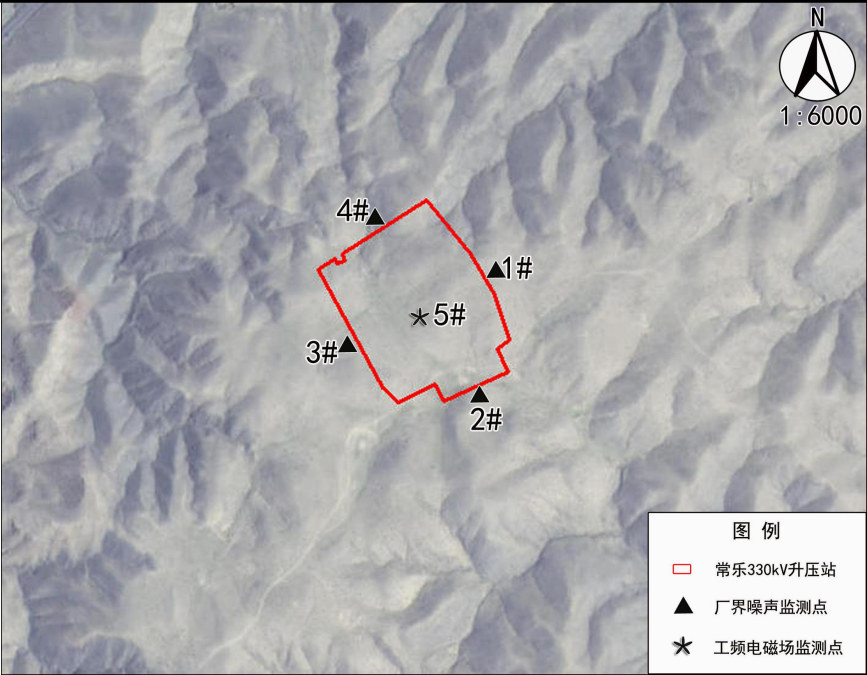
图 4.3-1 常乐升压站现状监测点位图
