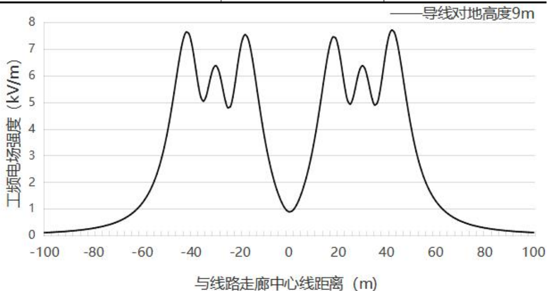
图 6.1-17 本项目线路与拟建永康~天都山 330kV 线路并行段工频电场强度变化趋势
