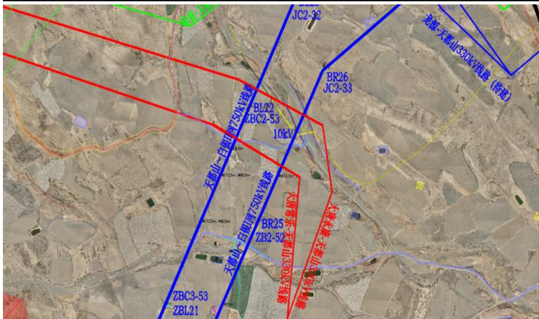
图 6.1-14 本项目交叉钻越线路示意图(1)
