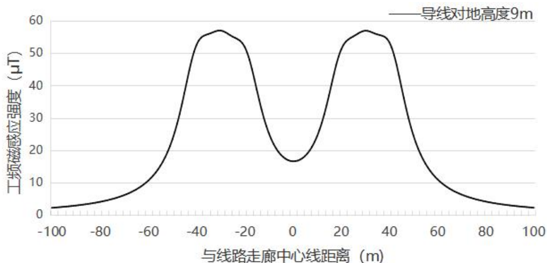
图 6.1-18 本项目线路与拟建常乐~天都山 330kV 线路并行段工频磁感应强度变化趋势
