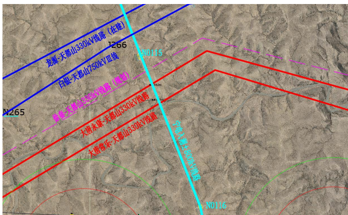
图 6.1-14 本项目交叉钻越及并行线路示意图(2)
