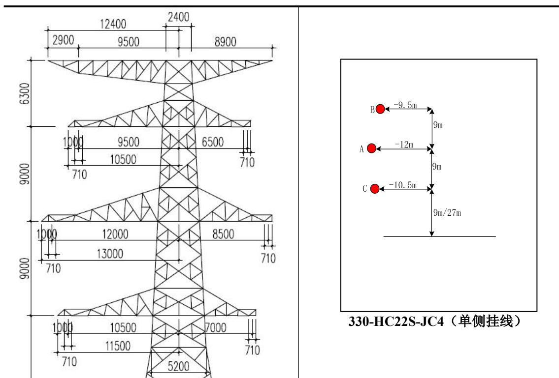
图 6.1-5 330kV 双回线路（单侧挂线）预测所选的塔型及预测参数示意图
