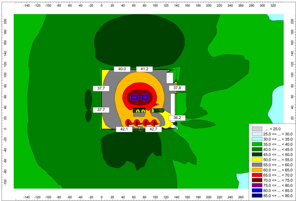
图 6.2-1 本项目升压站厂界噪声排放贡献值等声级线图
