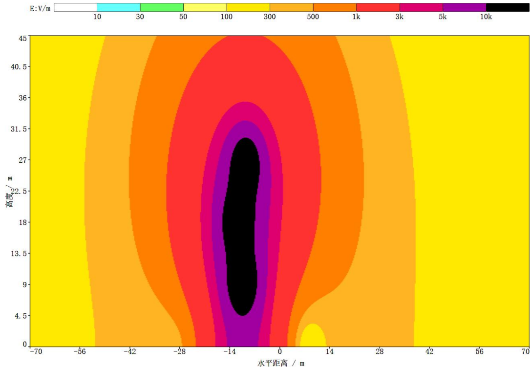
图 6.1-13 新建 330kV 双回线路（单侧挂线） 4\text{kV/m} 等值线图
